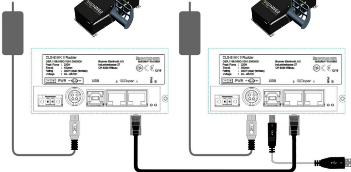
RJ-45 <= 3m
